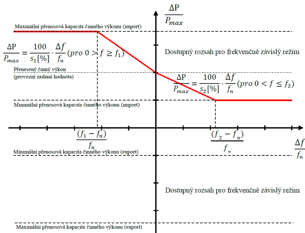
Obr. 2: Schopnost frekvenční odezvy činného výkonu u vysokonapěťové stejnosměrné soustavy ve frekvenčně závislém režimu na příkladu bez pásma necitlivosti a bez necitlivosti a s kladnou zadanou hodnotou činného výkonu (režim importu). \Delta P je změna činného výkonu na výstupu z vysokonapěťové stejnosměrné soustavy. f_n je cílová frekvence ve střídavé soustavě, ve které je služba frekvenčně závislého režimu poskytována, a \Delta f je odchylka frekvence ve střídavé soustavě, ve které je služba frekvenčně závislého režimu poskytována.
