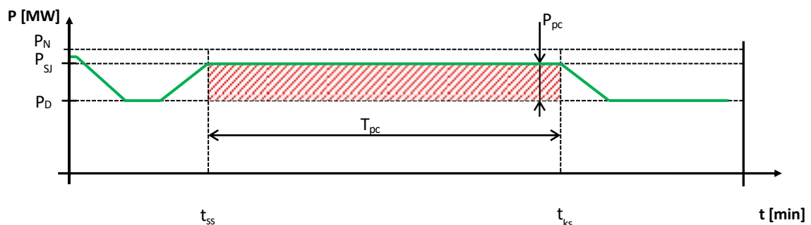
Obr. 13 Příklad smluvně sjednaných parametrů služby lokální stabilizace napětí
