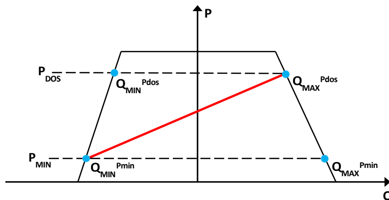
Obr. 8 Certifikovaný rozsah jalového výkonu
